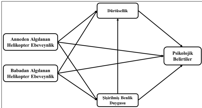
Şekil 1. Hipotetik Model
